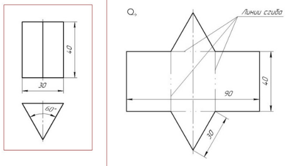
Развертка поверхностей правильной треугольной призмы представляет собой плоскую фигуру, составленную из боковых граней - прямоугольников и двух оснований - треугольников
